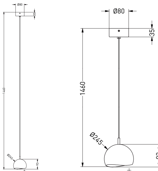
Technische tekening / Technical drawing
