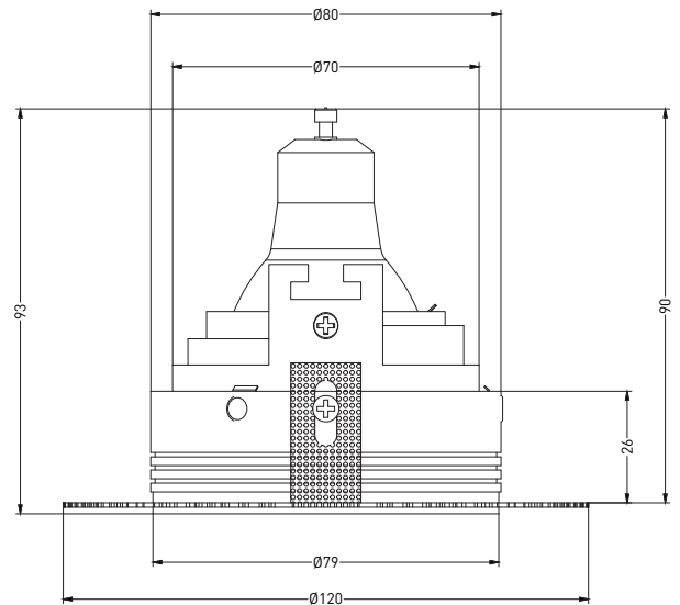
Technische tekening / Technical drawing
